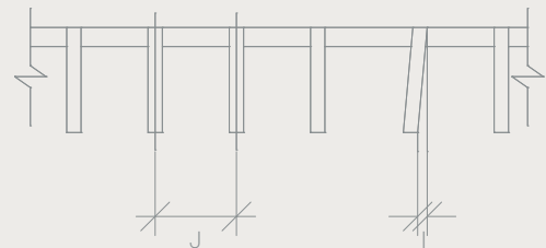
Schrägstellung der Trag- und Randstäbe I \max. = 0,1 \times J , jedoch max. 3 mm
