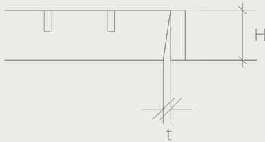
Schrägschnitt des Tragstabes bzw. Querstabes t \max. = \pm 0,1 \times H , jedoch max. 3 mm
