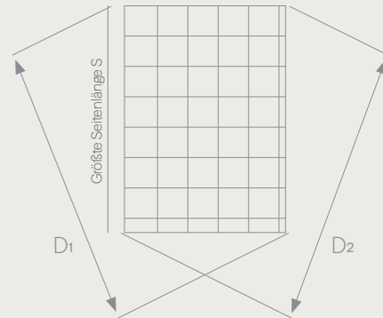
Diagonalverzug : D1-D2 \leq 0,01 \times s
