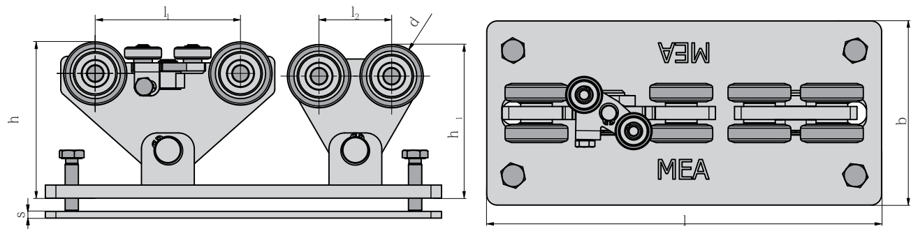
Laufrolle FRT Nr. 3
