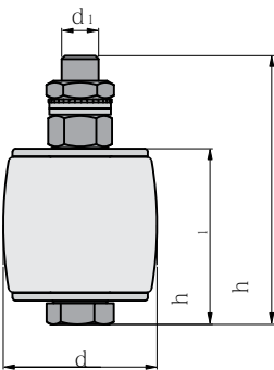
Außenführungsrolle, Nylon, lose
