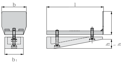
Auflaufkeil Stahl/Nylon
