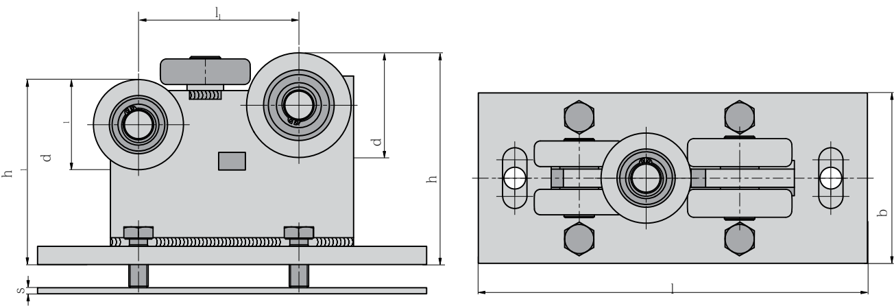
Laufrolle FRT Nr. 5
