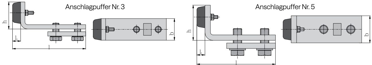
Anschlagpuffer, galvanisch verzinkt
