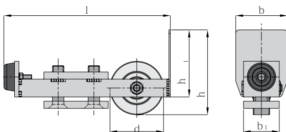
Auflaufrolle, galvanisch verzinkt, inklusive Anschlagpuffer
