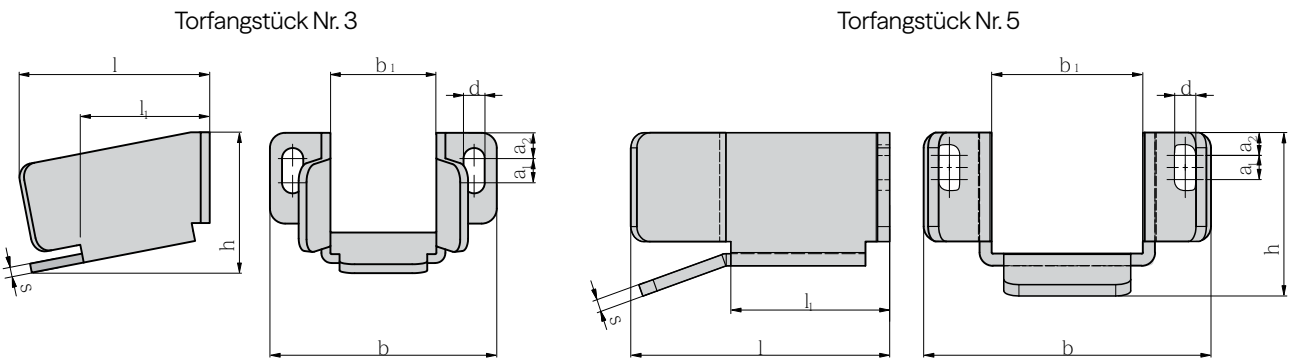
Torfangstück, galvanisch verzinkt
