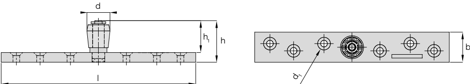
Bodenführungsrolle Nylon mit Platte
