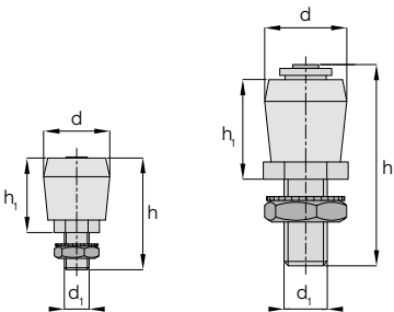
Bodenführungsrolle Nr. 19
