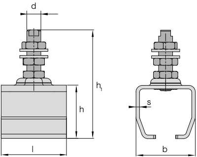
Muffe, für Höhen- und Seitenverstellung
