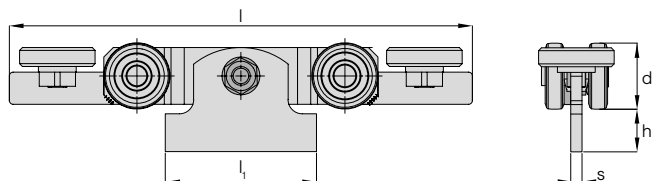
Doppelrolle mit Seitenführung und Anschweißpendel
