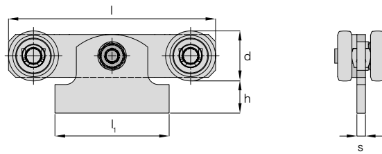
Doppelrolle mit Anschweißpendel
