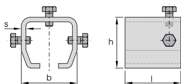
Schweißmuffe unverzinkt oder galvanisch verzinkt
