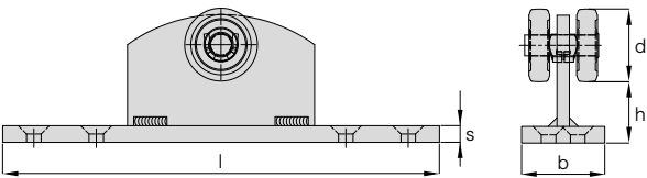
Einfachrolle mit Flansch
