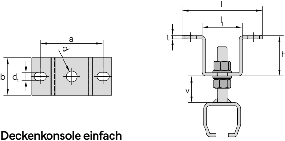
Deckenkonsole einfach
