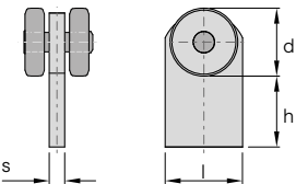
Einfachrolle zum Anschweißen
