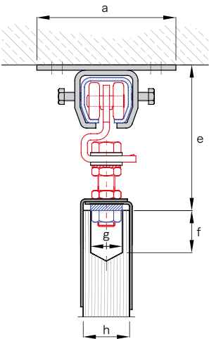
Deckenbefestigung
