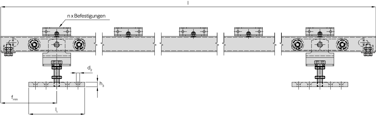
Komplettsortiment Größe Nr. 0 – für Türgewichte bis zu 75 kg
