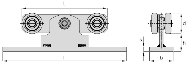
Doppelrolle mit Flanschpendel
