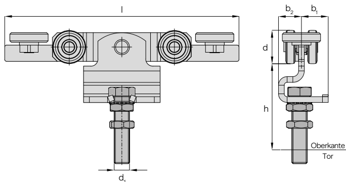
Doppelrolle mit Seitenführung und Sechskantschraube
