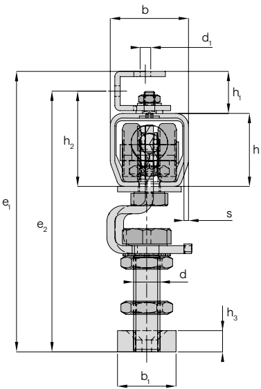
Anschlussmaße
