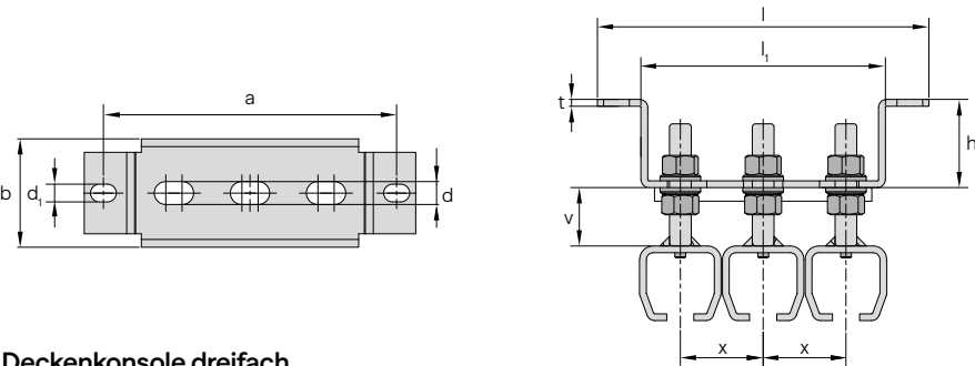
Deckenkonsole dreifach
