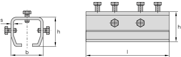
Verbindungsmuffe
