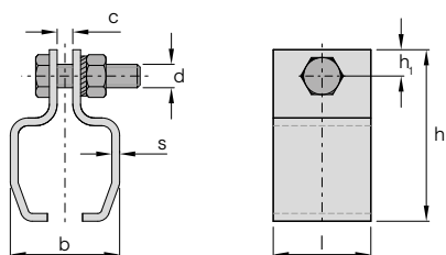
Aufhängeklemme
