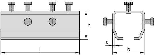
Verbindungsmuffe
