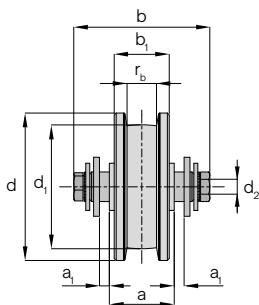
Stahlrolle unten doppelt gelagert
