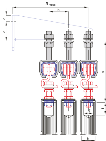
Wandkonsole dreifach mit H/S-Muffen
