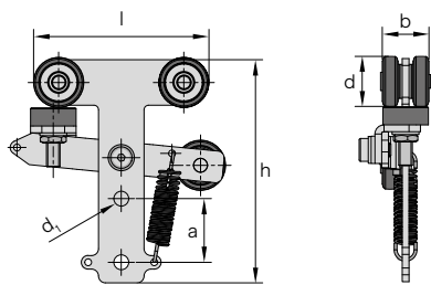
Doppelrolle mit Stopper
