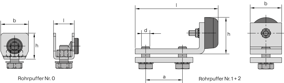
Rohrpuffer
