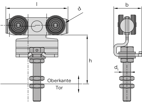
Doppelrolle, mit Kunststoffrollen
