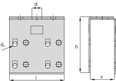
Verstärkungslasche
