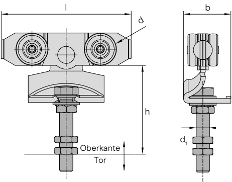
Doppelrolle
