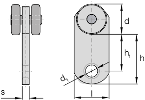
Einfachrolle zum Einhängen
