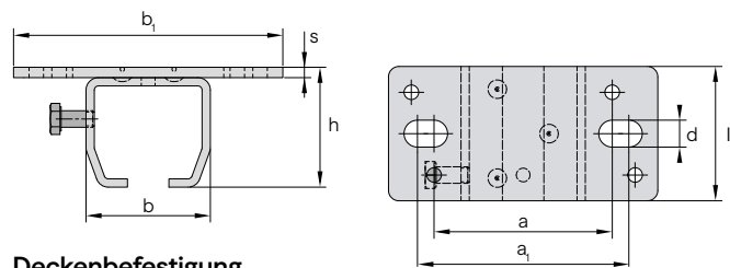
Deckenbefestigung
