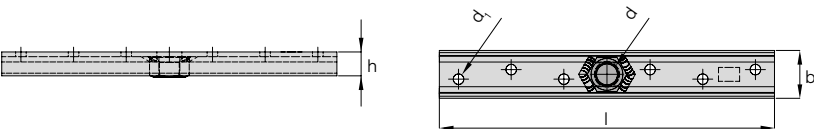
Trägerplatte
