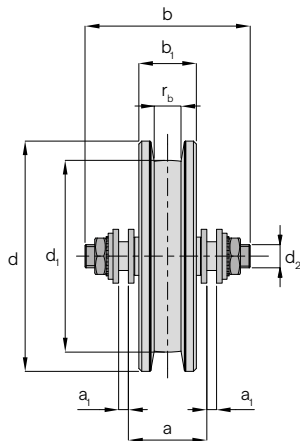
Stahlrolle unten einfach gelagert
