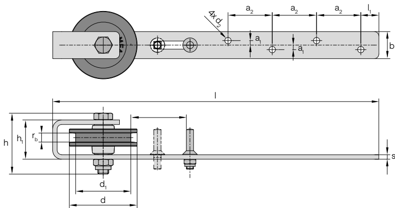
MEA Gussrollen mit galvanisch verzinktem Bügel
