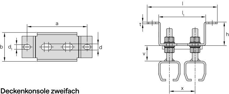
Deckenkonsole zweifach
