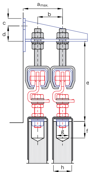
Wandkonsole zweifach mit H/S-Muffen
