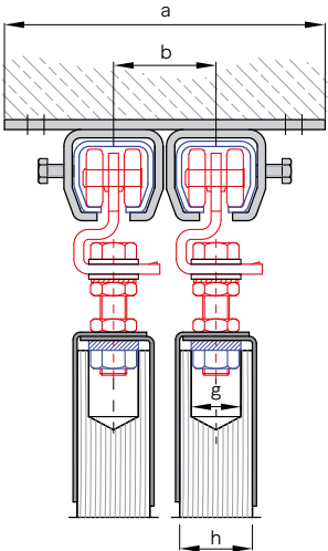
Doppeldeckenbefestigung
