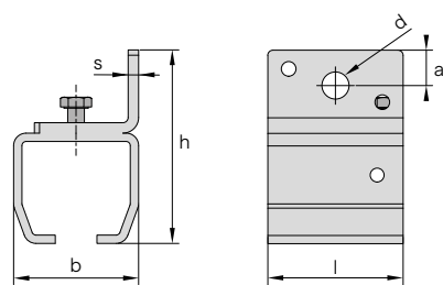
Wandbefestigung
