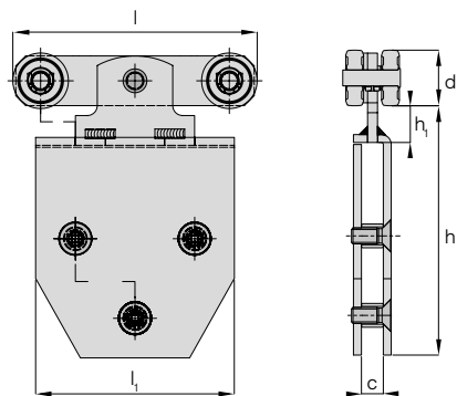
Doppelrolle, für Platten
