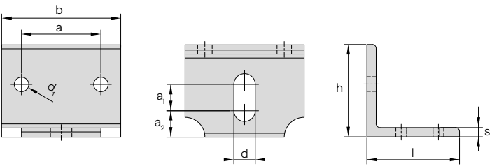
Einfachkonsole
