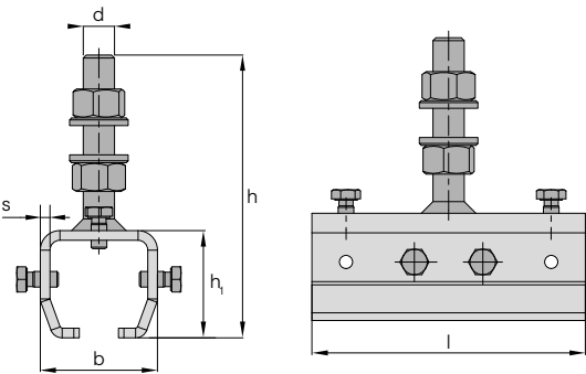
Verbindungsmuffe H/S verstellbar
