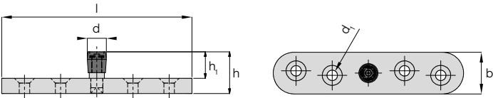
Bodenführungsrolle Messing mit Platte
